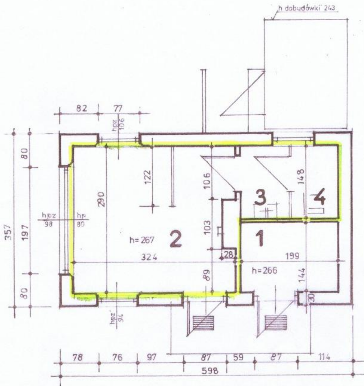
RZUT PRZYZIEMIA 1:50
